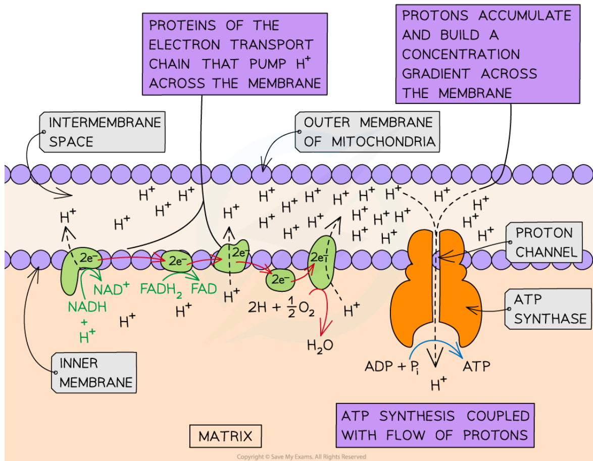
Chemiosmosis Diagram
